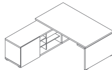
MITF2L 1800-2078 / 2080 / 740 237.4 kg
