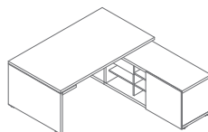
MIT1P 2000-2278 / 2080 / 740 230.05 kg
