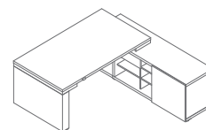
MIT2RP 1990 / 2080 / 1300-760 348.3 kg
